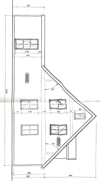
ZIJGEVEL LINKS - SCHAAAL 1/50
