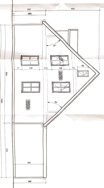
ZIJGEVEL RECHTS - SCHAAAL 1/50
