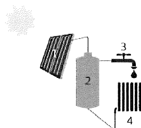
1. Zonnecollector | 2. Opslagvat zonneboiler | 3. Sanitair warm water | 4. Afjijfelement voor ruimteverwarming (inplueneel)
